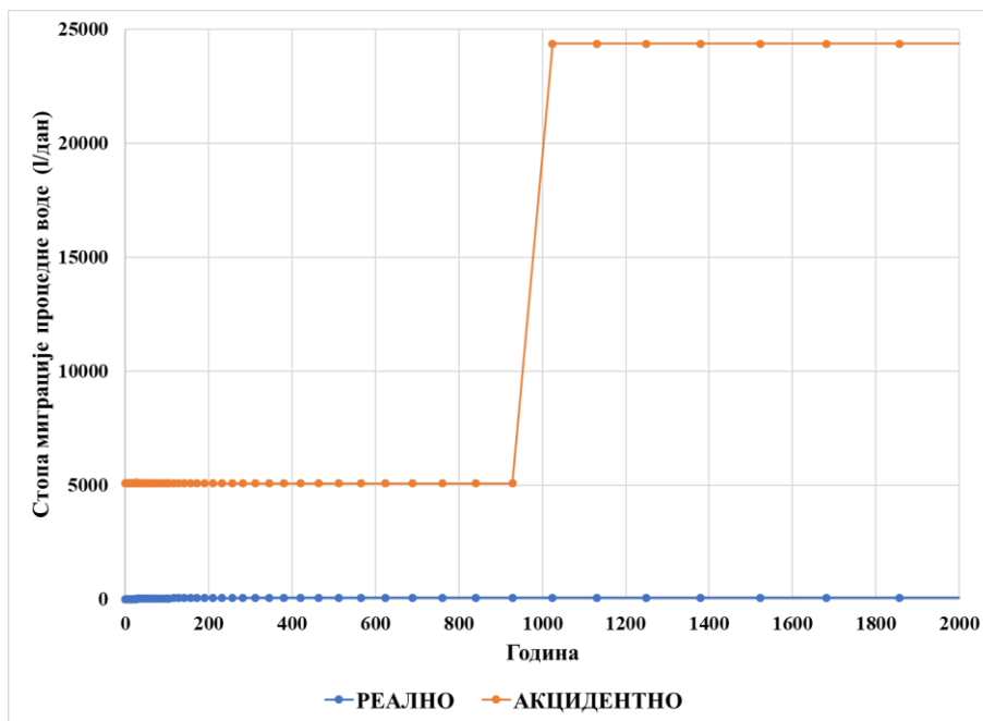
Слика 8.33 Стопа миграције проведне воде на моделу реалног и акцидентног стања депоније „Гигош“
